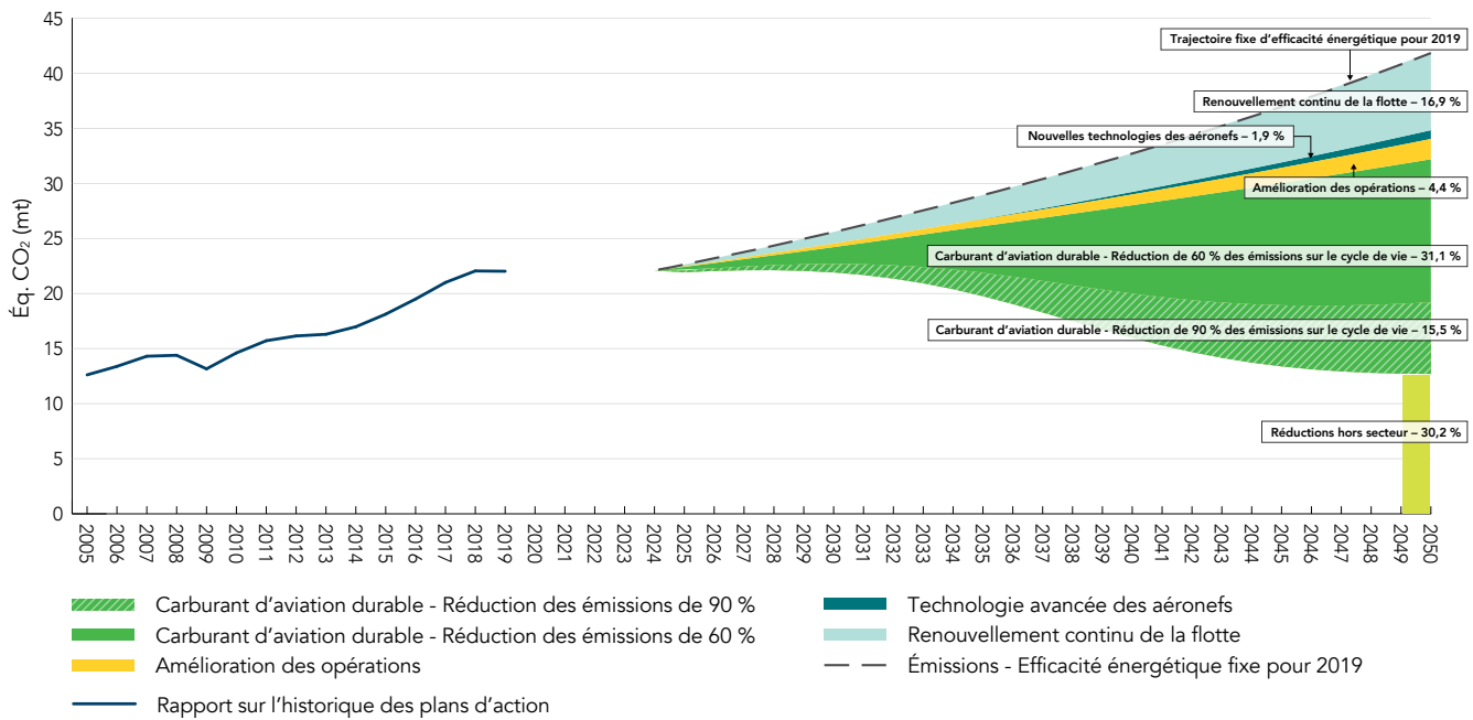
GRAPHIQUE 2. Prévisions des émissions des aéronefs canadiens en 2050 – Une vision vers la carboneutralité
